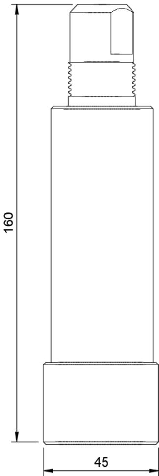
Rysunek 1: Wymiary sondy SH-45w
